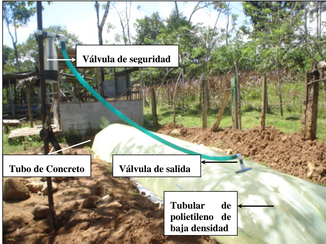
Figura 2. Partes de un biodigestor tipo Taiwán (Polietileno de baja densidad)
