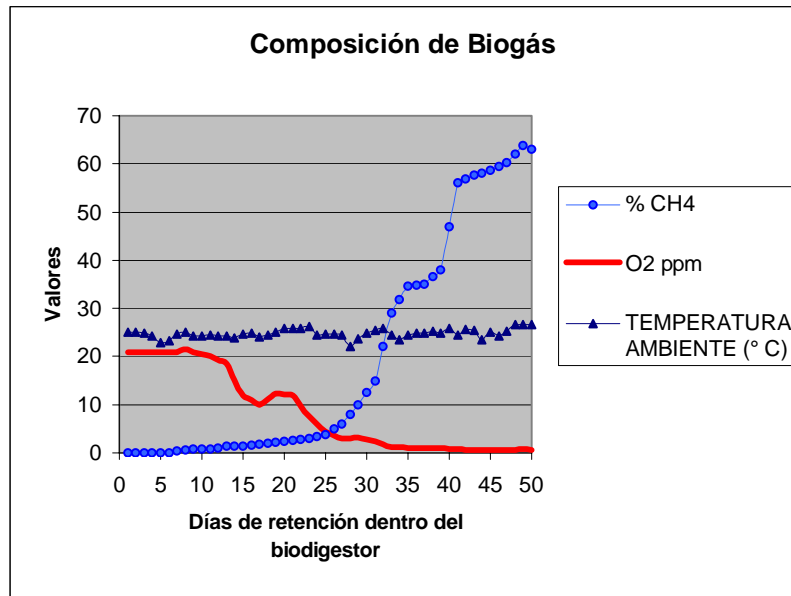
Figura 11. Composición del biogás obtenido de la Unidad de cerdos de Zamorano.
