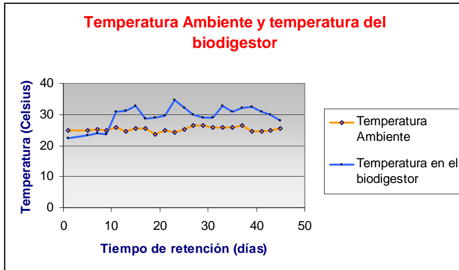
Figura 12. Temperatura ambiente Vs temperatura dentro del biodigestor
