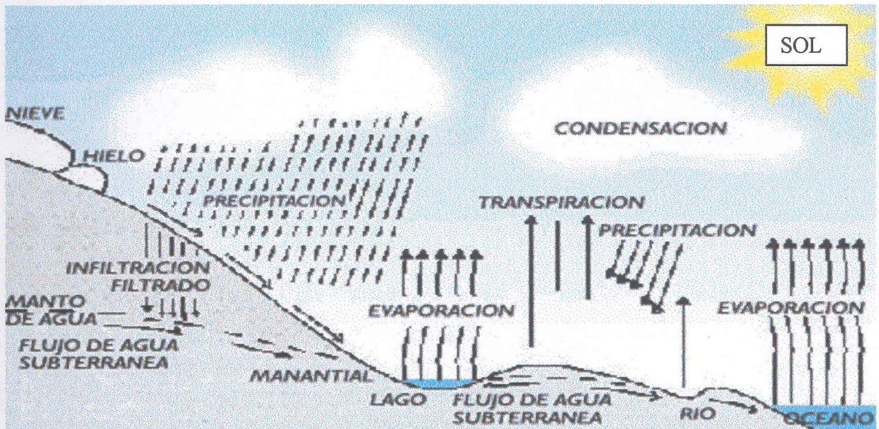
Figura 1. Ciclo hidrológico.
