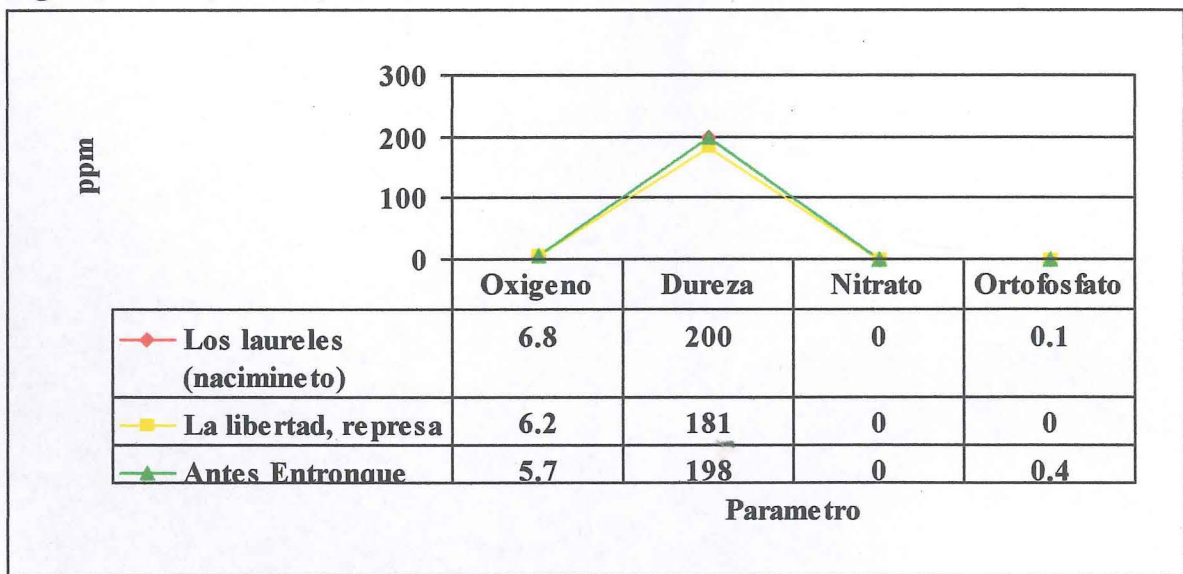
Niveles de oxígeno, dureza, nitrato y ortofosfato durante el mes de agosto en tres sitios de la microcuenca del río Salitroso municipio de La Libertad, Honduras 2001
