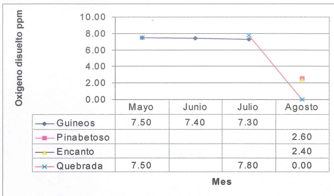
Figura 12 Niveles de oxígeno disuelto en cada sito por mes para la microcuenca El Encanto, Comayagua, Honduras.
